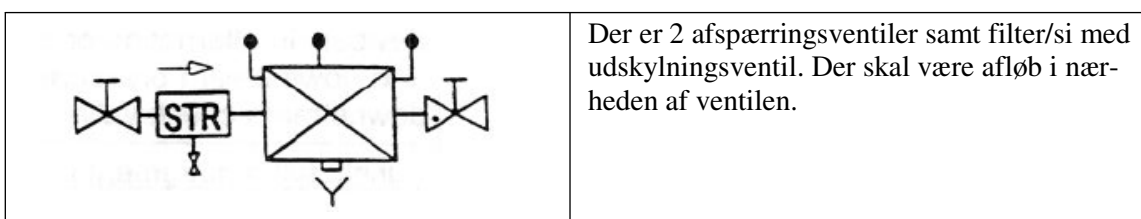
Figur 5.8 Installationskravet til en tilbagestrømningsventil af typen
